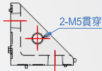
加工型(封板用孔)
