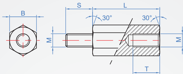
鐵材導角30°
