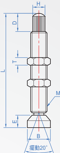
B：活動頭
